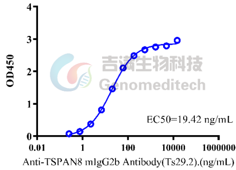
Fig. ELISA
