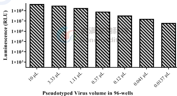
图2 吉满 SARS-CoV-2 Spike S 蛋白(JN.1.11.1)突变型假病毒感染 HEK293T-ACE2 测定 Luciferase 数值
